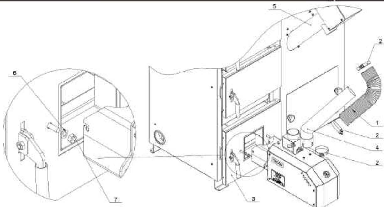
Рис. 7 Установка пеллетной горелки TECO PELLET
