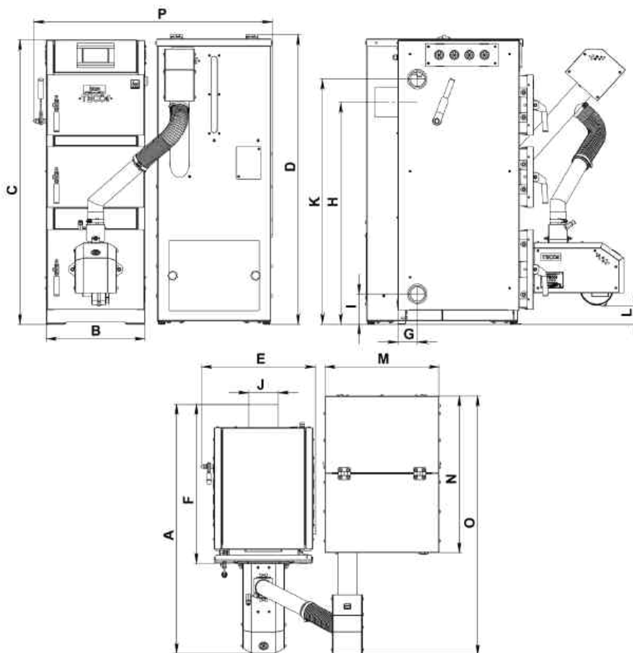
Рис. 1 Основные размеры котла
