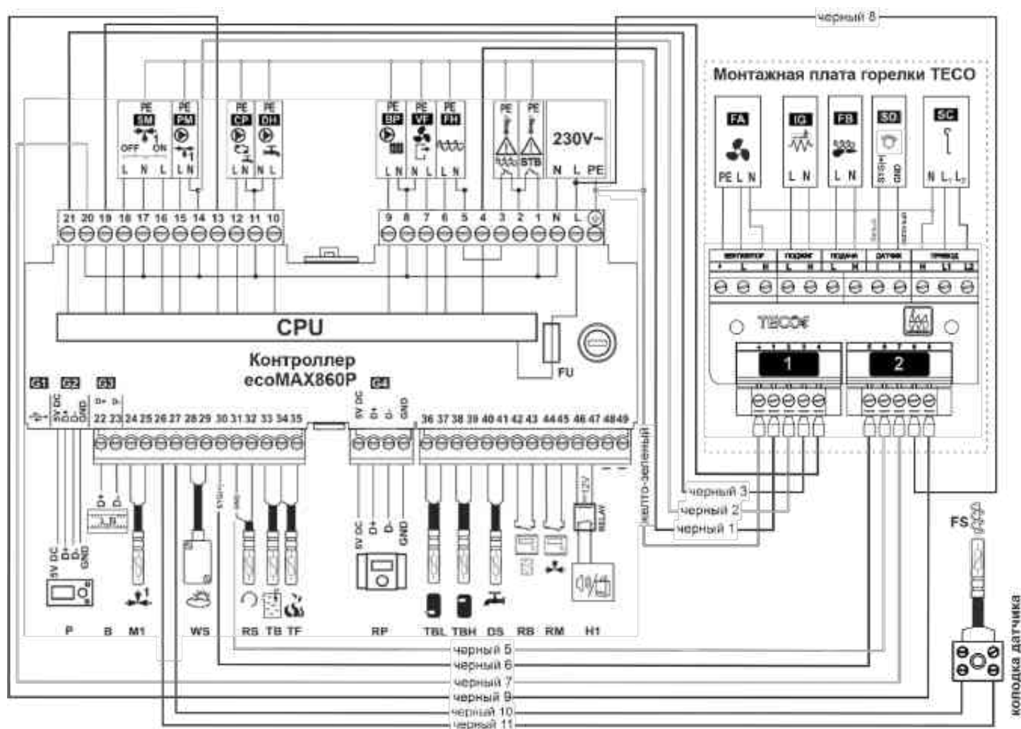
Рис. 8 Схема электрического подключения пеллетной горелки TECO PELLET
