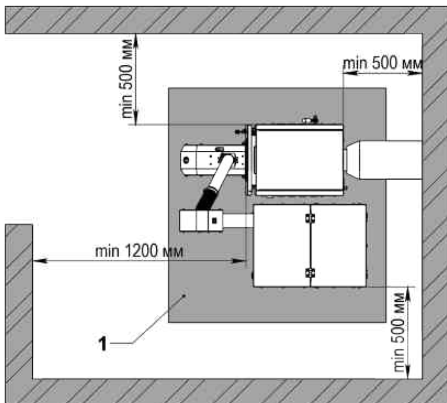
Рис. 12 Установка котла
