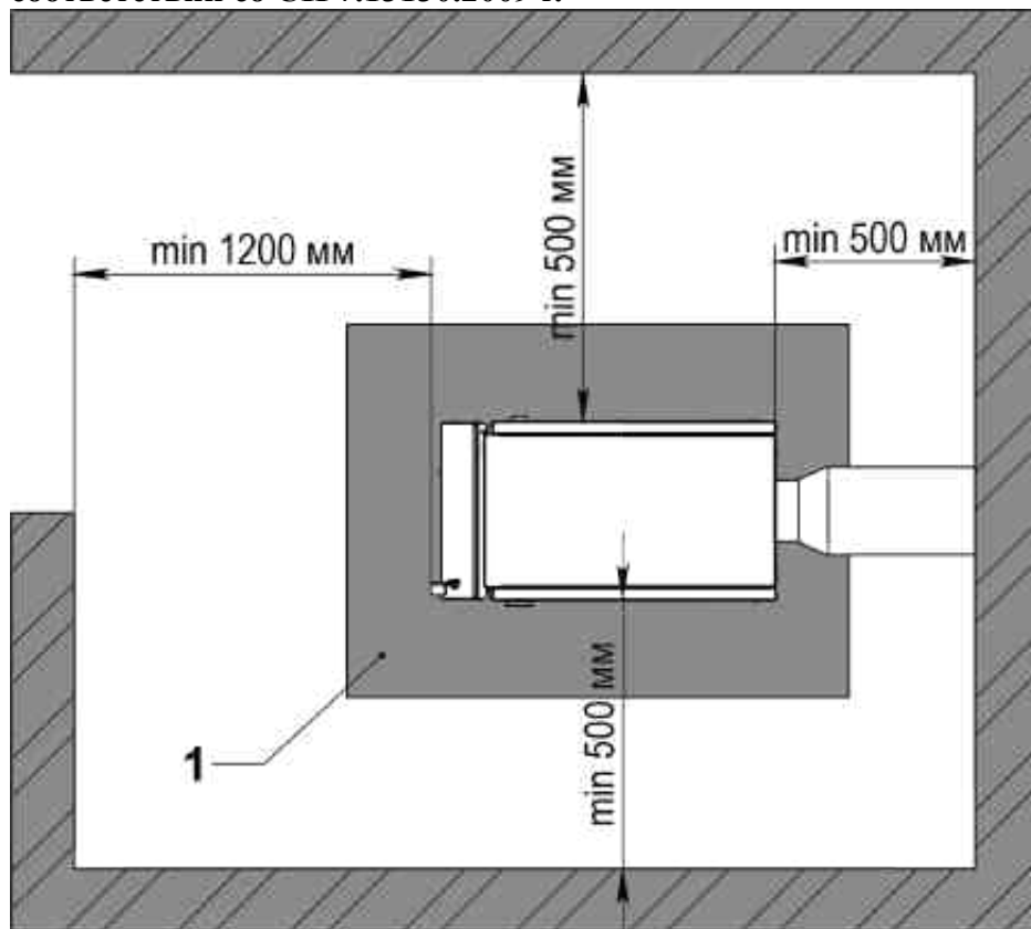
Рис. 7 Установка котла
