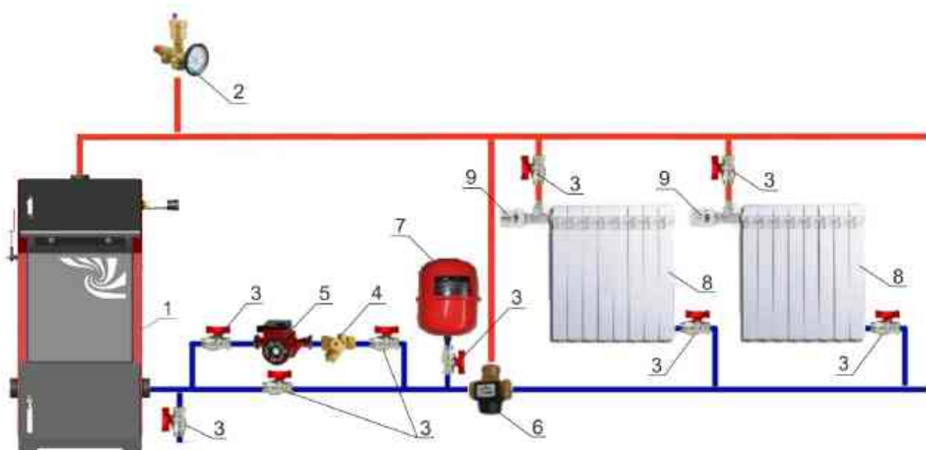
Рис. 10 Схема подключения котла к закрытой системе с принудительной циркуляцией теплоносителя с термостатическим смесительным клапаном 1
