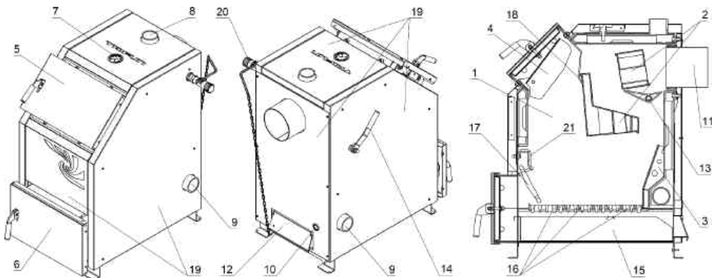
Рис. 3 Устройство котла TAIFUN 20 кВт
