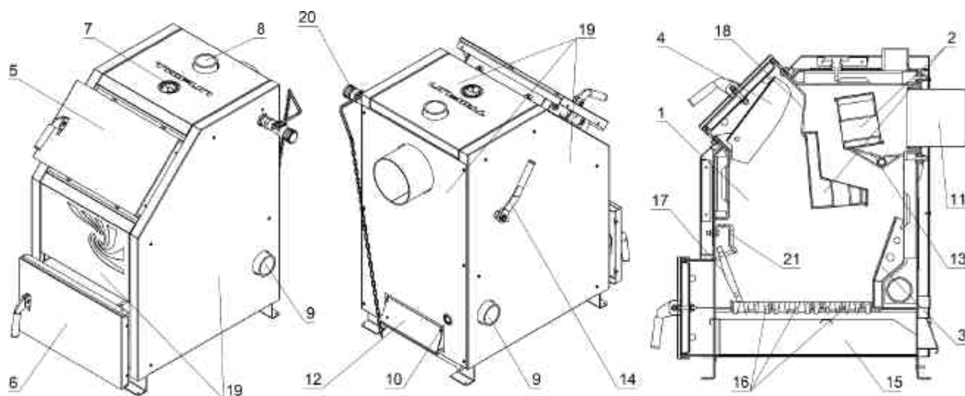
Рис. 2 Устройство котла TAIFUN 16 кВт
